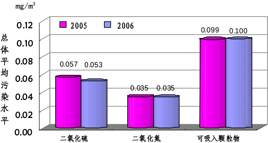
重点城市主要污染物年均浓度
