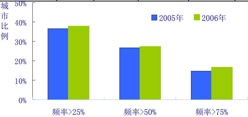
不同酸雨频率城市比例
