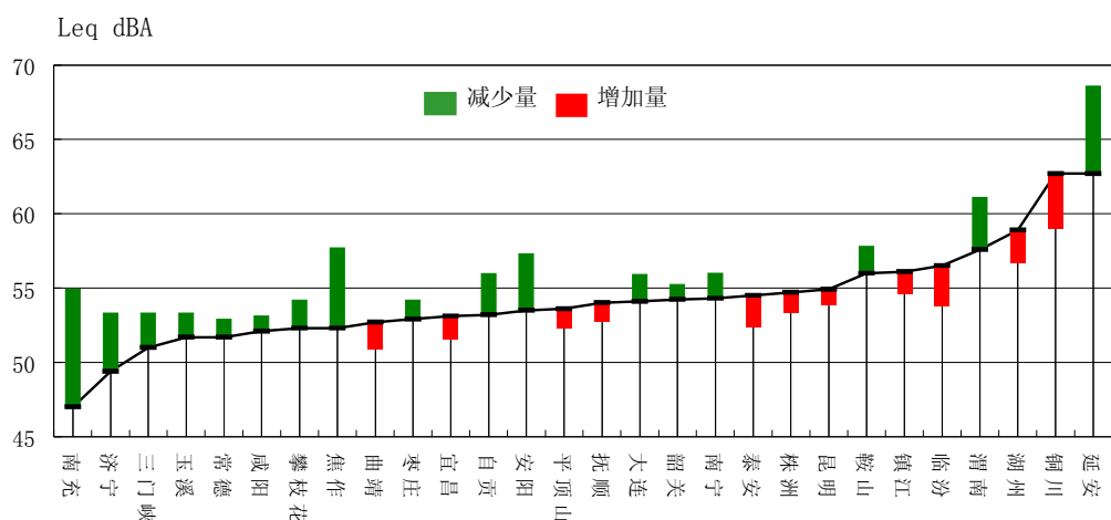
(所列为变化幅度等于或超过 1dB ( A ) 的城市) 2006 年重点城市区域环境噪声等效声级与上年比较
