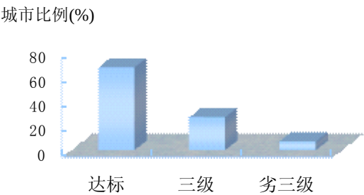
2006 年颗粒物浓度分级城市比例
