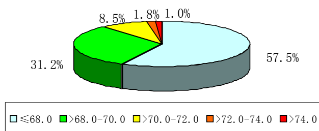
2006 年城市道路交通声环境质量状况
