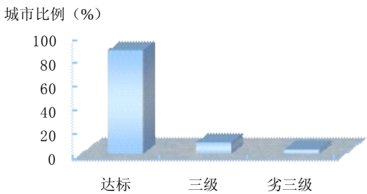
2006 年二氧化硫浓度分级城市比例
