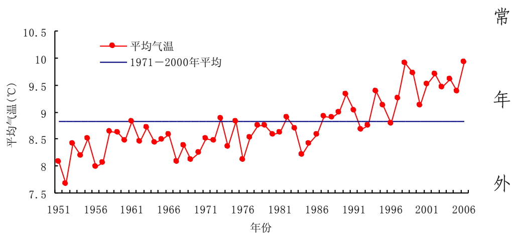
全国年平均气温历年变化 ( ^{\circ}\text{C} )
