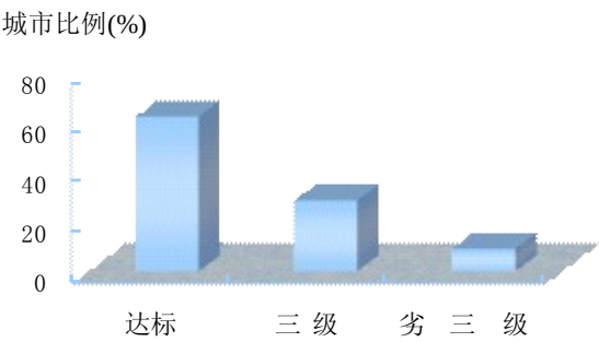
2006 年城市空气质量级别比例
