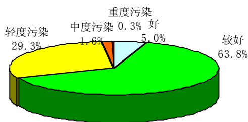
2006 年城市区域声环境质量状况
