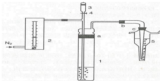
图 19-1 硫化物测定的吹气装置
