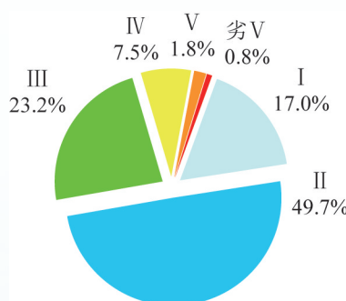
图 1-3 2022 年 2 月全国主要江河水质类别比例
