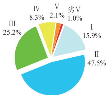
图 1-1 2022 年 2 月全国地表水水质类别比例
