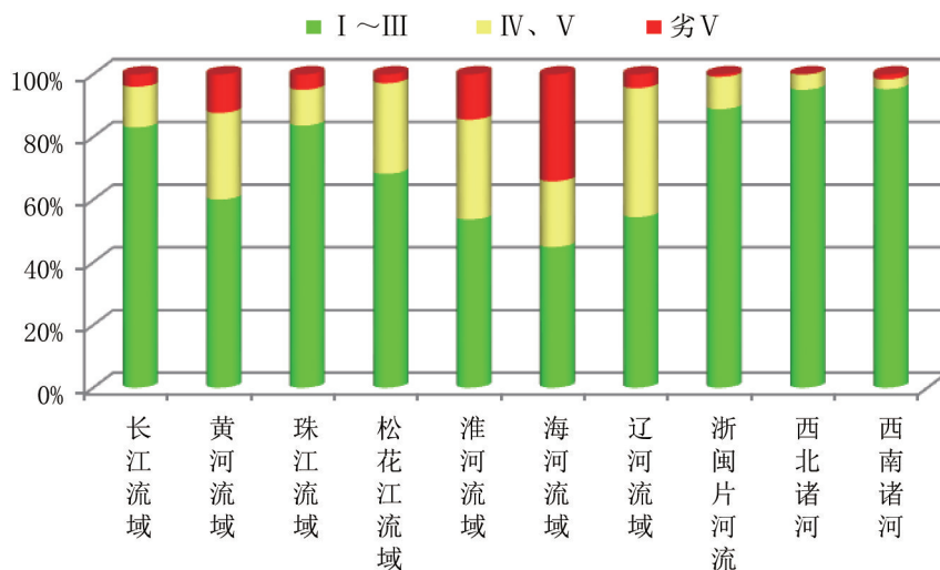
图1-3 2016年7月十大流域水质类别比例
