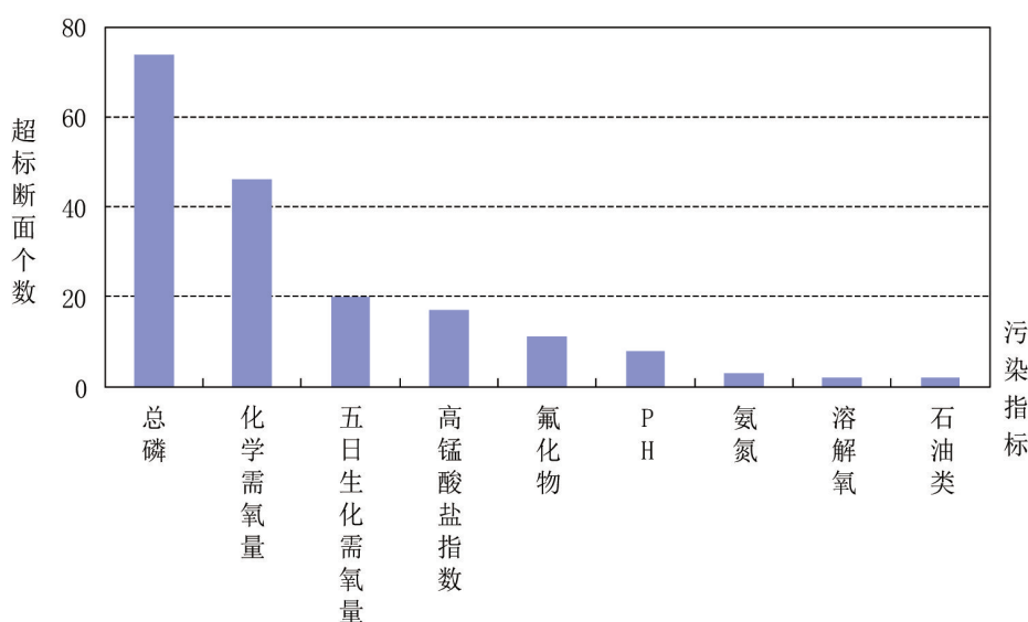
图1-4 2016年7月全国重点湖库污染指标统计
