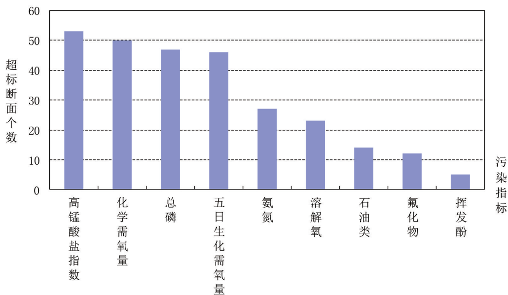
图2-9 淮河流域水体污染指标统计
