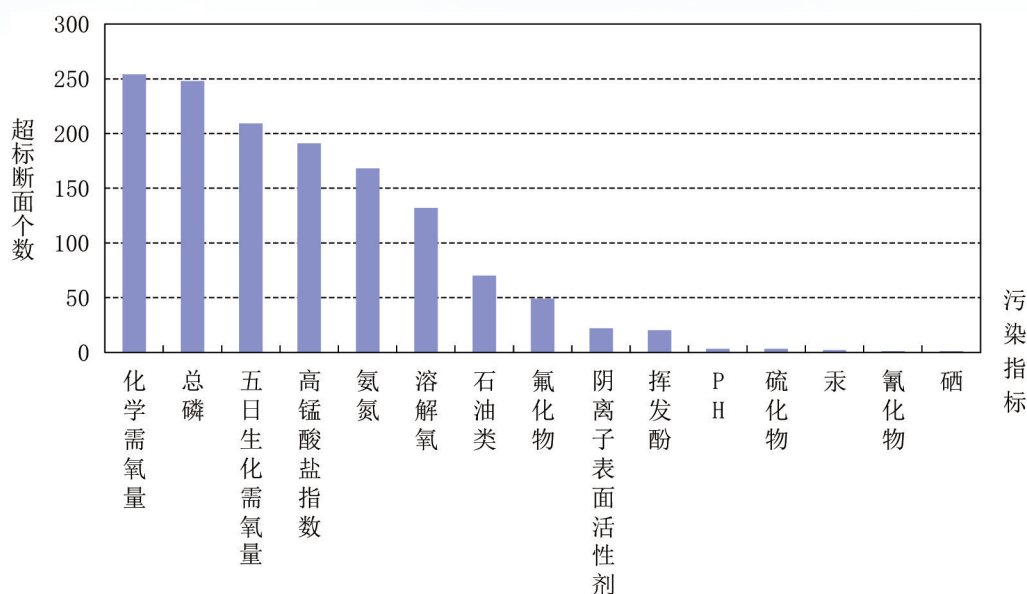
图1-2 2016年7月全国主要江河水系污染指标统计
