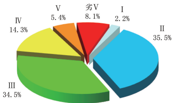
图 1-1 2016 年 7 月全国主要江河水系水质类别比例
