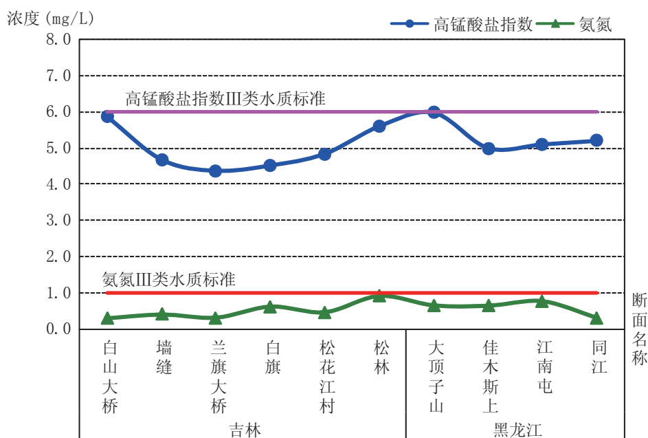
图2-12 松花江干流高锰酸盐指数、氨氮沿程变化
