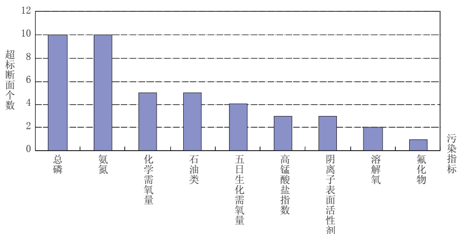
图2-1 长江流域水体污染指标统计
