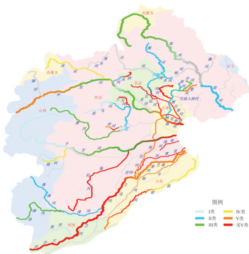
图2-17 2013年12月海河流域水质分布示意图
