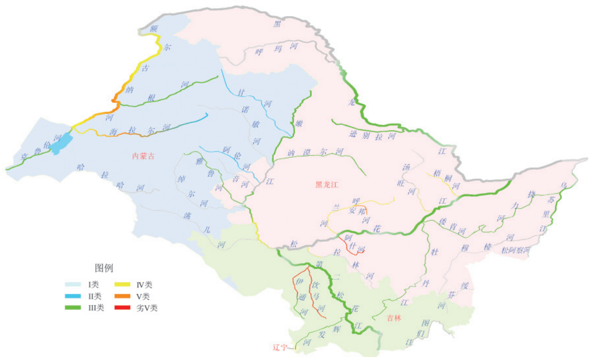
图2-11 2013年12月松花江流域水质分布示意图
