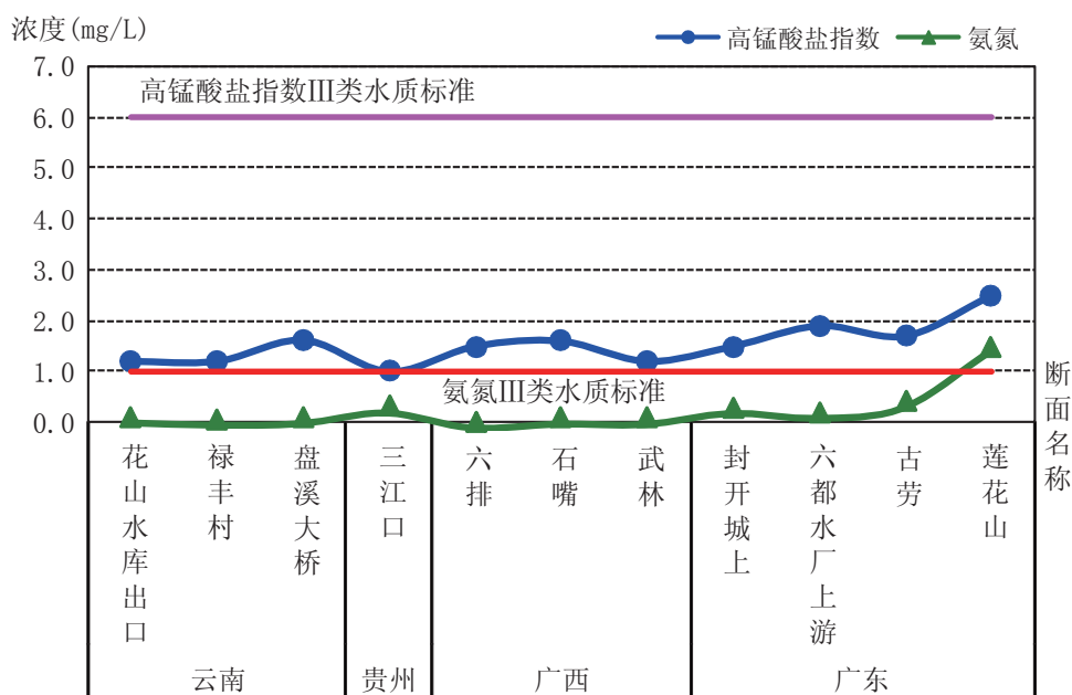
图2-9 珠江干流（西江）高锰酸盐指数、氨氮沿程变化
