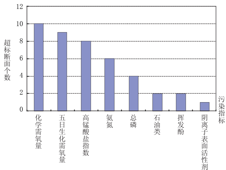
图2-10 松花江流域水体污染指标统计
