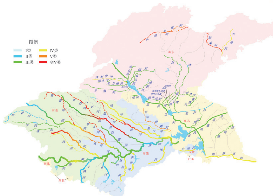
图2-14 2013年12月淮河流域水质分布示意图
