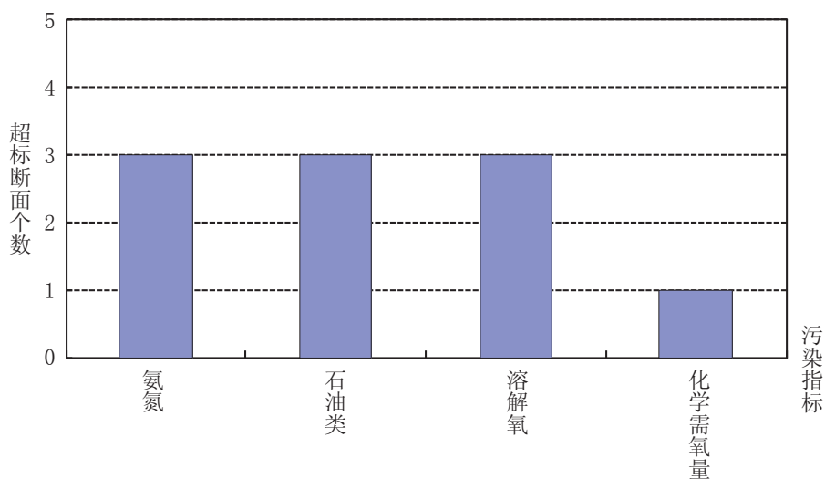
图2-21 浙闽片河流污染指标统计
