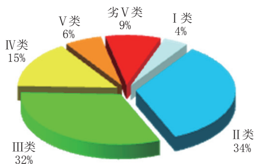
图1-1 2013年12月全国主要江河水系水质类别比例
