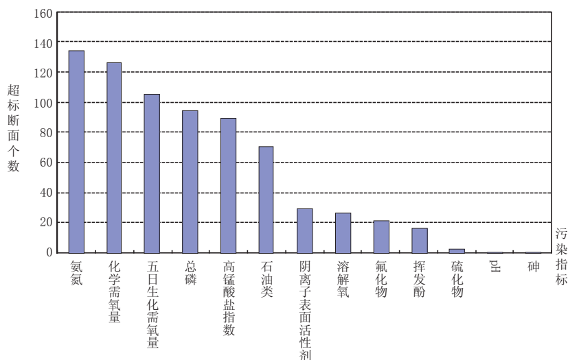
图1-2 2013年12月全国主要江河水系污染指标统计
