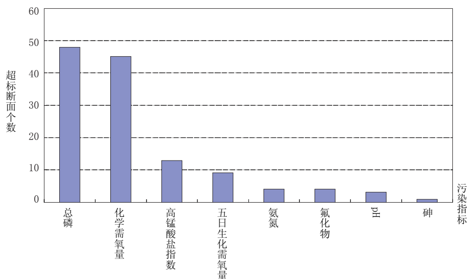
图1-4 2013年12月全国重点湖库污染指标统计
