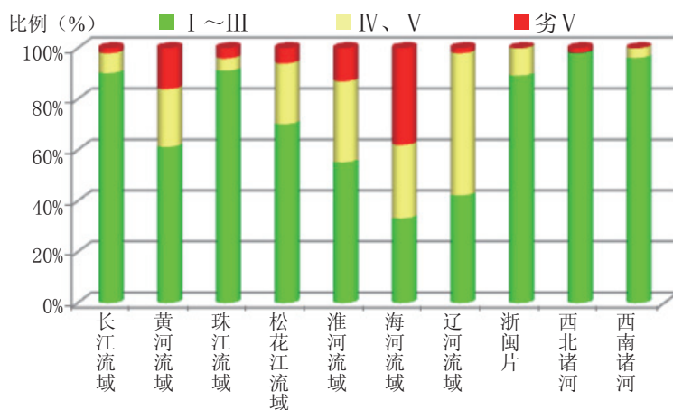
图1-3 2013年12月十大流域水质类别比例
