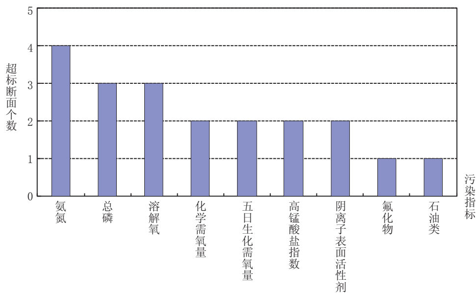
图2-7 珠江流域水体污染指标统计
