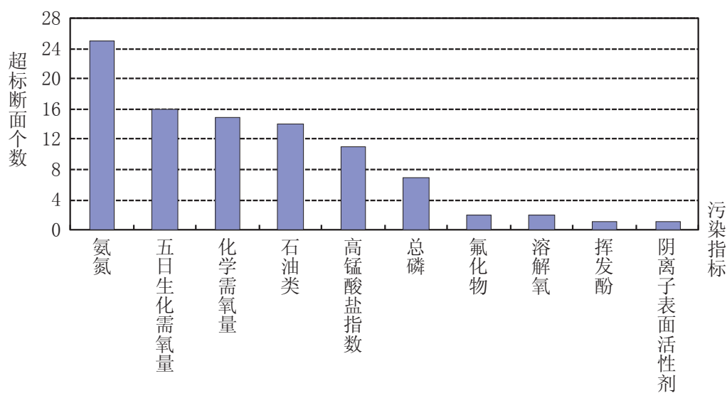
图2-18 辽河流域水体污染指标统计
