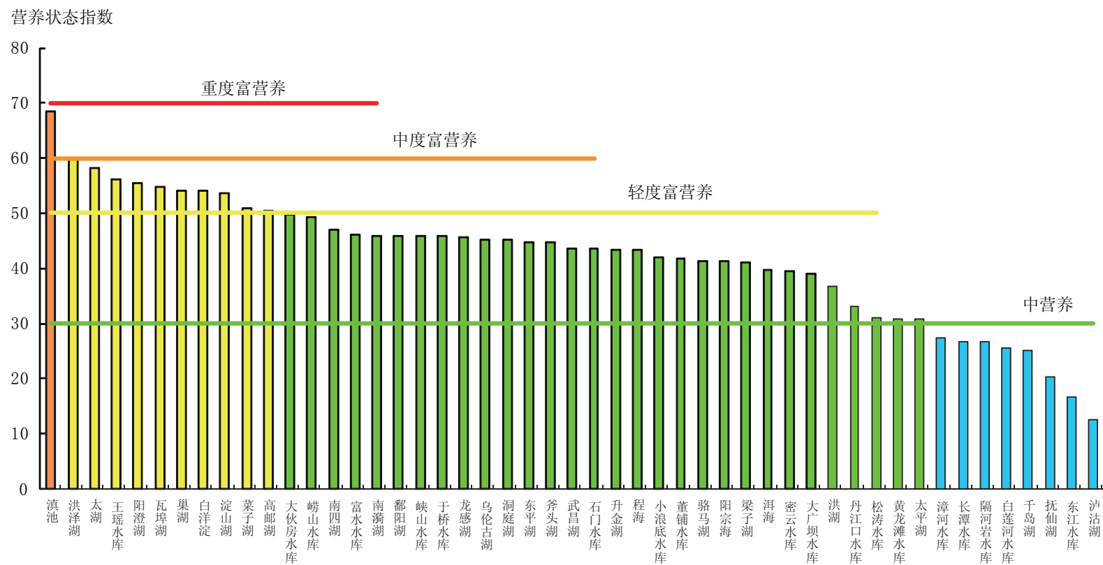
图 1-5 2013年12月全国重点湖库营养状态指数比较
