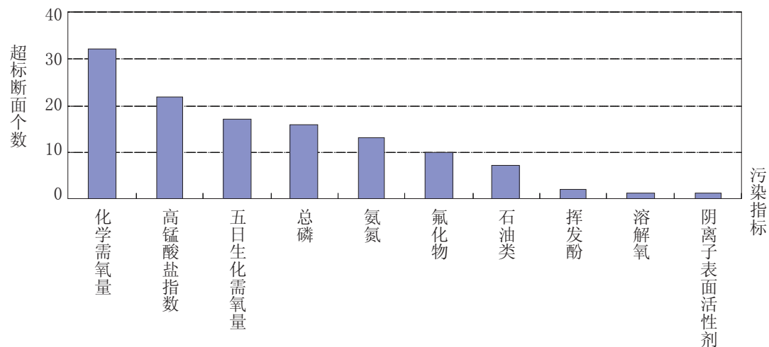
图2-13 淮河流域水体污染指标统计
