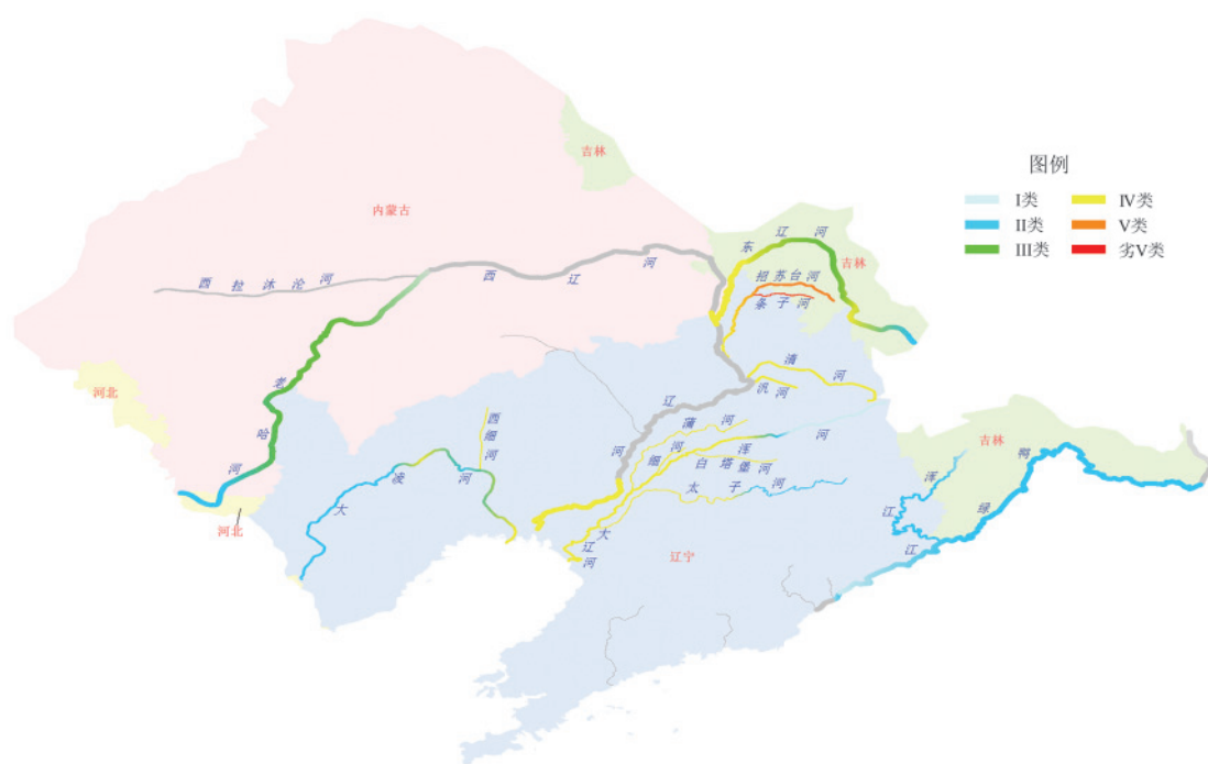
图2-19 2013年12月辽河流域水质分布示意图
