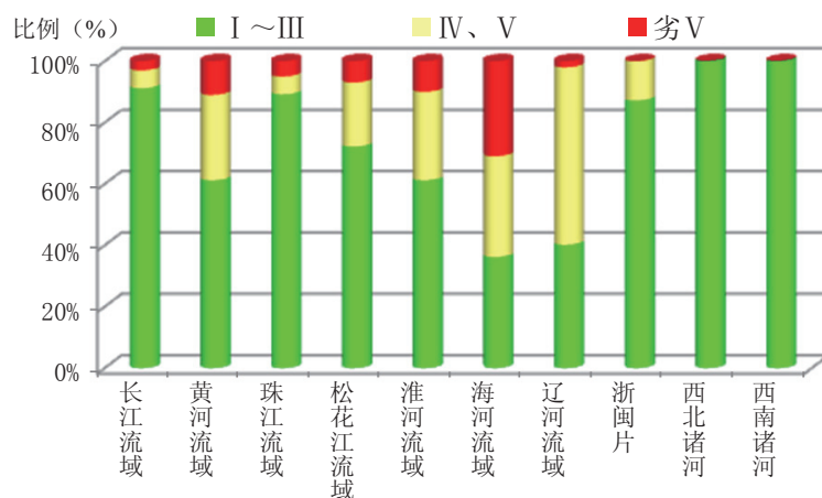
图1-3 2013年11月十大流域水质类别比例
