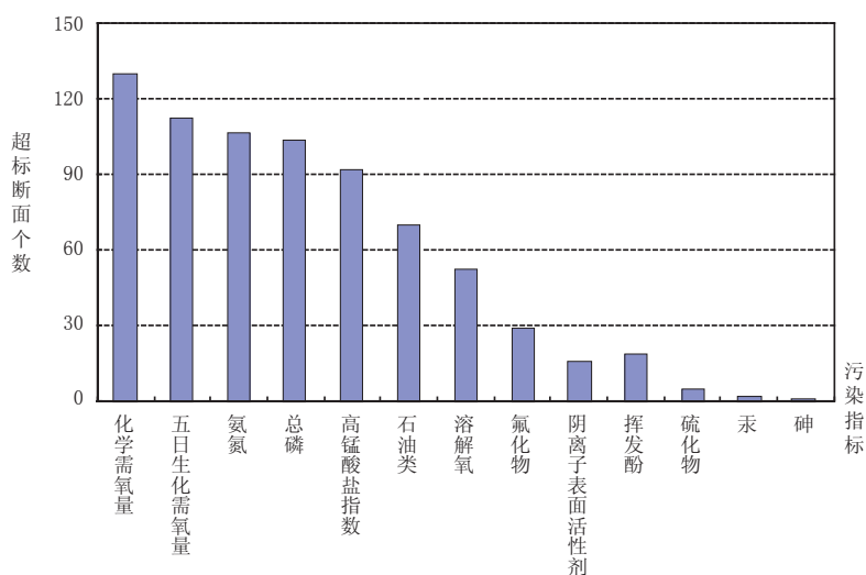
图1-2 2013年11月全国主要江河水系污染指标统计
