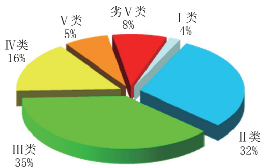
图1-1 2013年11月全国主要江河水系水质类别比例
