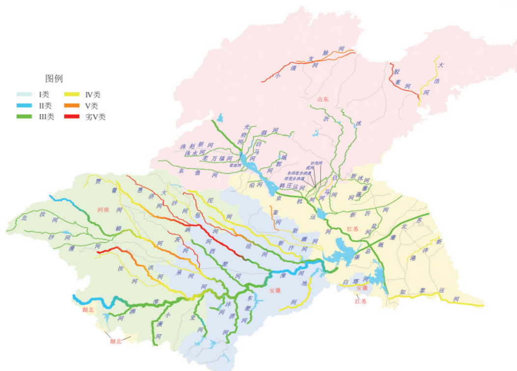
图2-14 2013年11月淮河流域水质分布示意图
