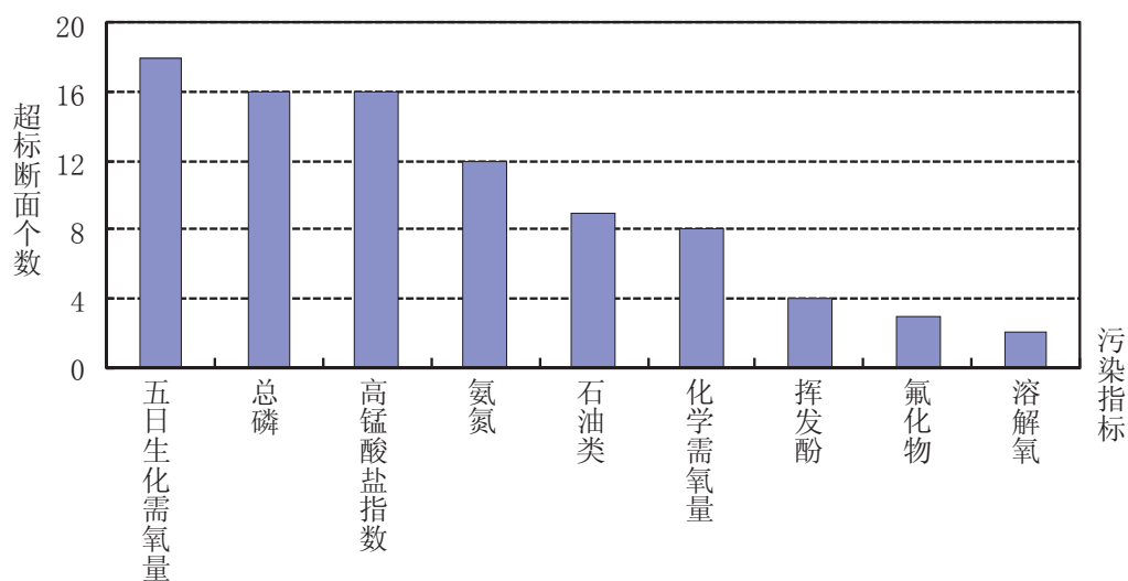
图2-18 辽河流域水体污染指标统计
