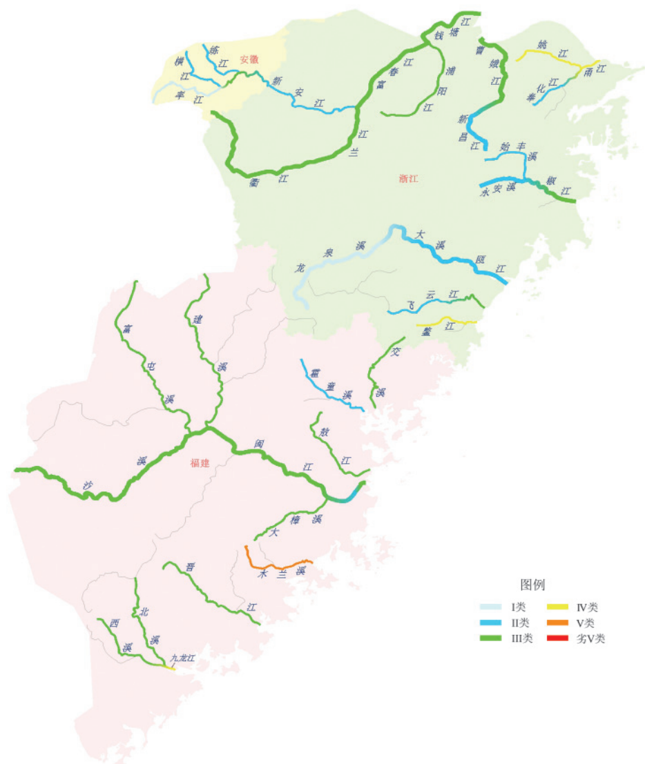
图2-22 2013年11月浙闽片河流水质分布示意图
