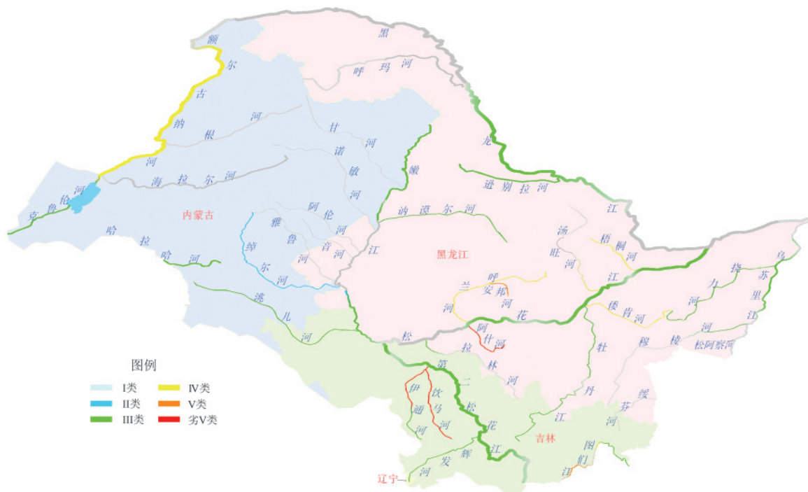
图2-11 2013年11月松花江流域水质分布示意图
