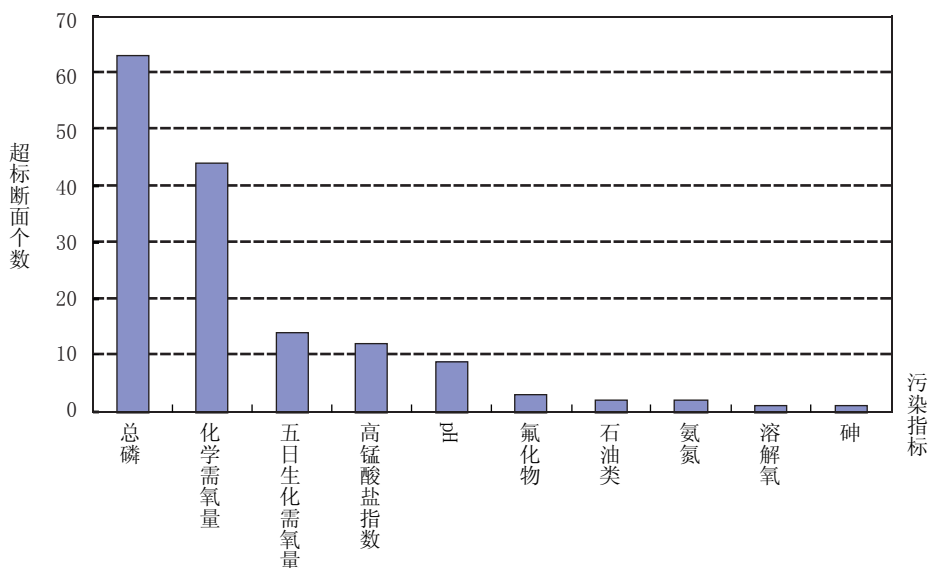
图1-4 2013年11月全国重点湖库污染指标统计
