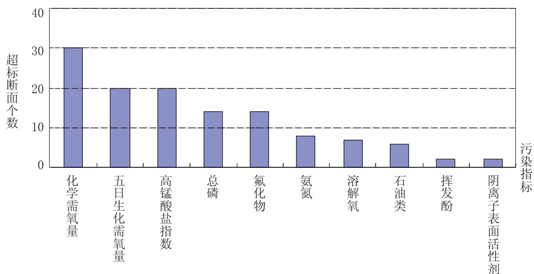
图2-13 淮河流域水体污染指标统计
