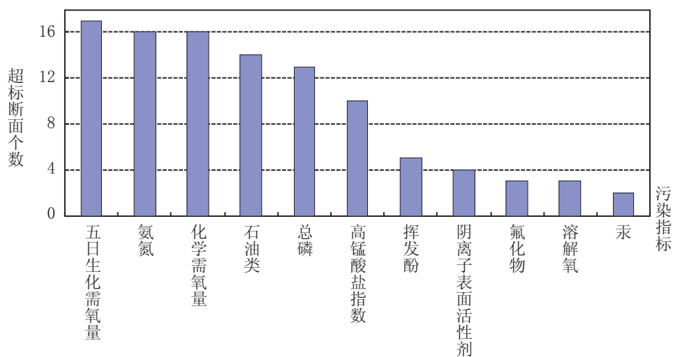
图2-4 黄河流域水体污染指标统计
