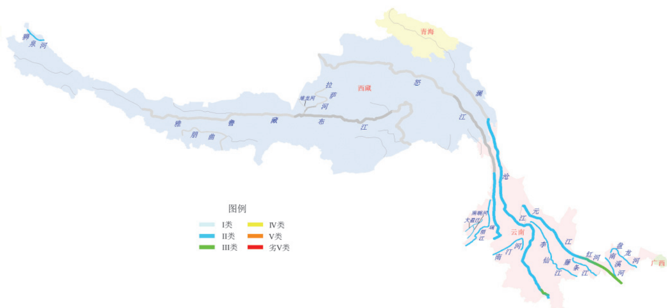
图2-24 2013年10月西南诸河河流水质分布示意图
