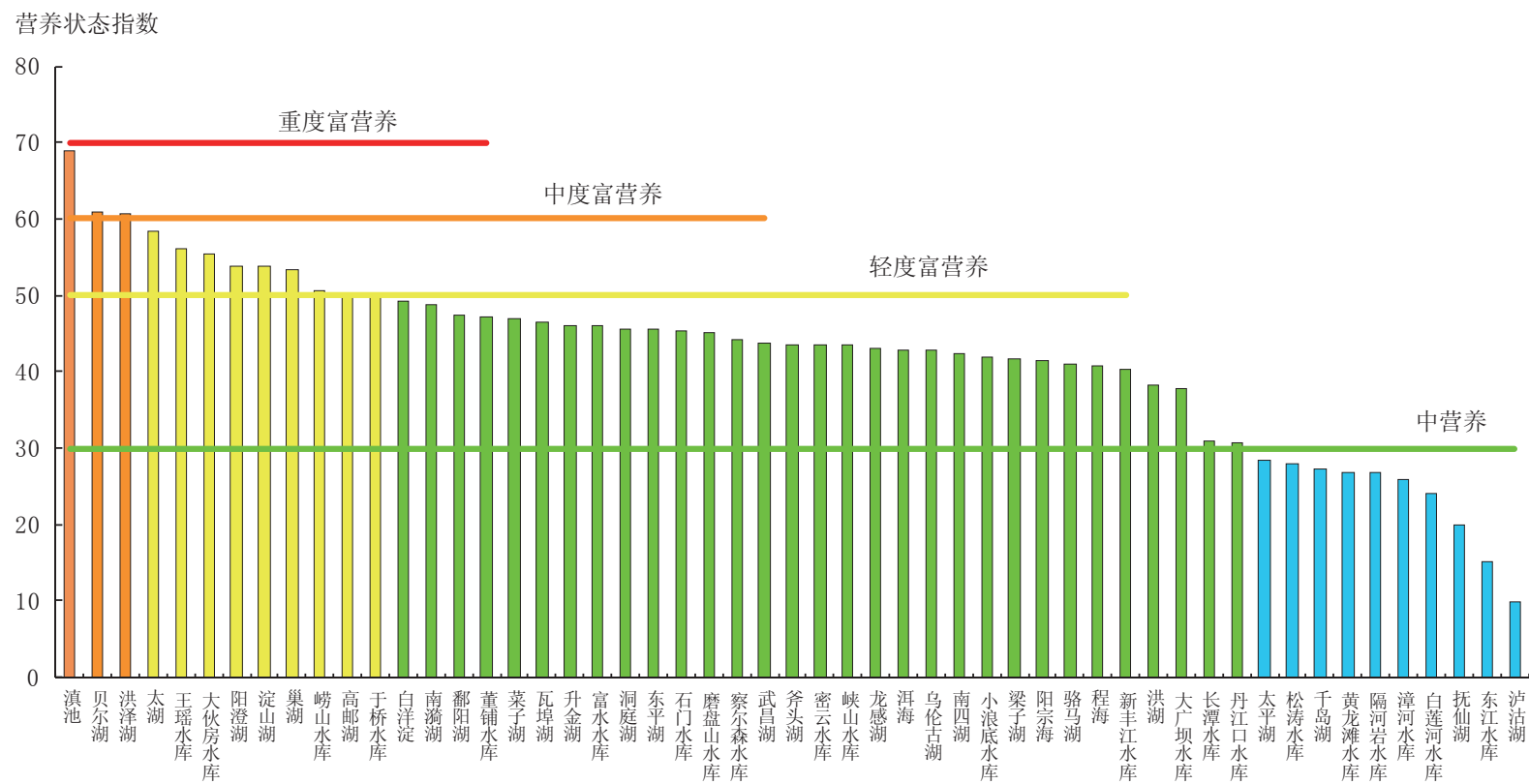
图 1-5 2013年11月全国重点湖库营养状态指数比较
