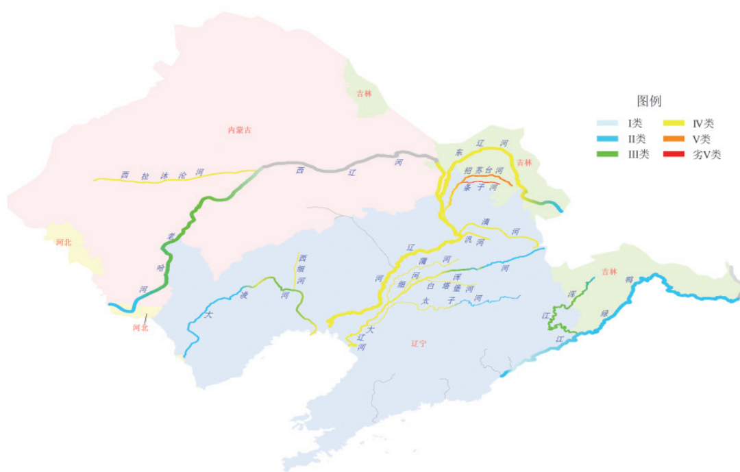
图2-19 2013年11月辽河流域水质分布示意图
