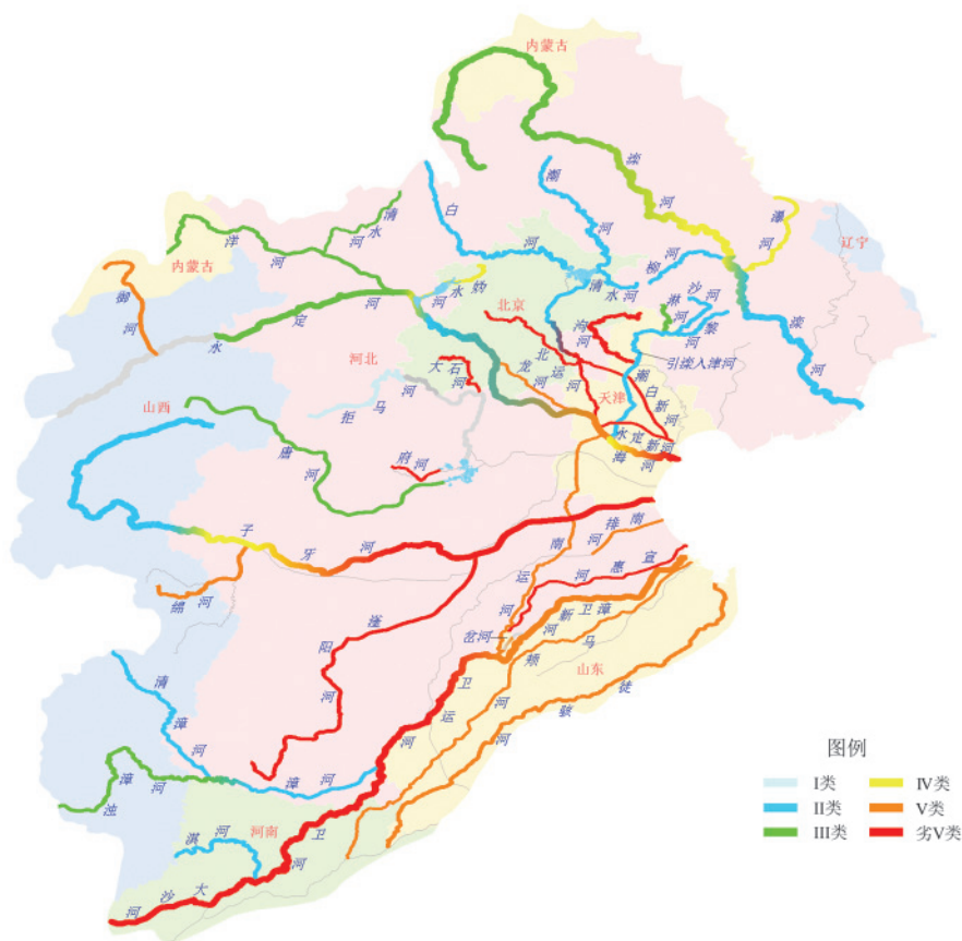
图2-17 2013年11月海河流域水质分布示意图
