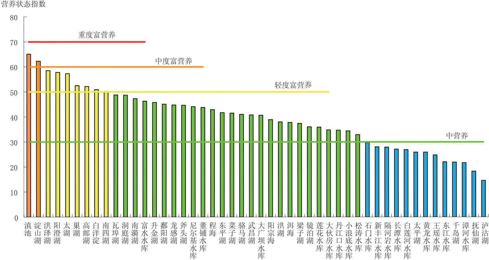
图 1-5 2013年2月全国重点湖库营养状态指数比较
