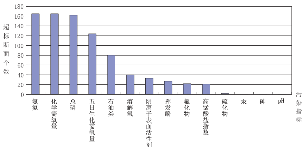
图1-2 2013年2月全国主要江河水系污染指标统计
