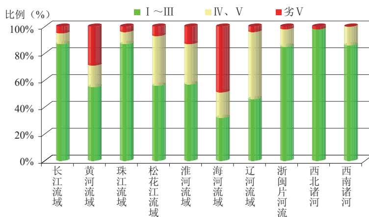
图1-3 2013年2月十大流域水质类别比例
