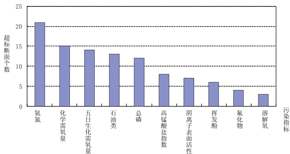
图1-4 2013年2月全国重点湖库污染指标统计
