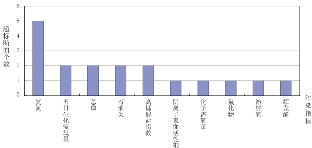
图2-5 珠江流域水体污染指标统计
