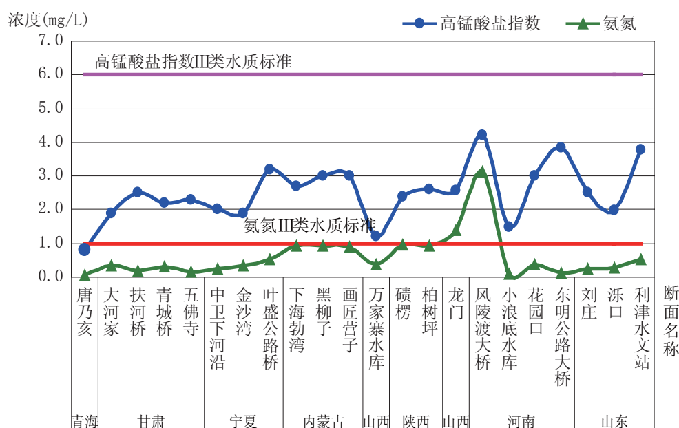
图2-4 黄河干流高锰酸盐指数、氨氮沿程变化
