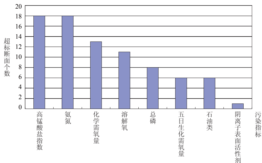
图2-7 松花江流域水体污染指标统计
