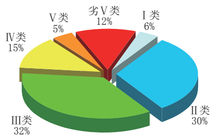
图1-1 2013年2月全国主要江河水系水质类别比例
