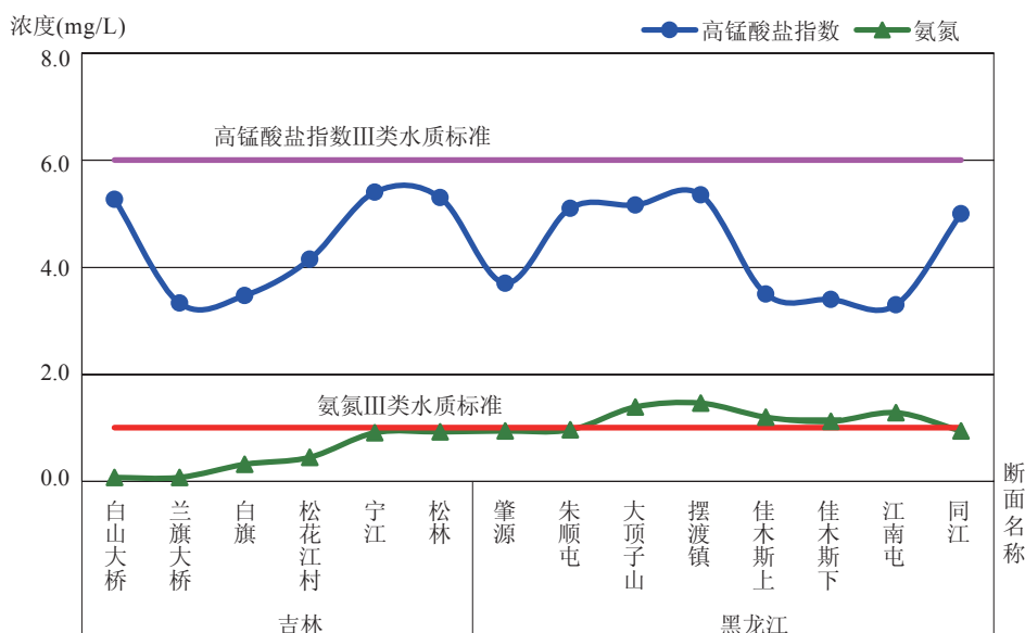
图2-8 松花江干流高锰酸盐指数、氨氮沿程变化
