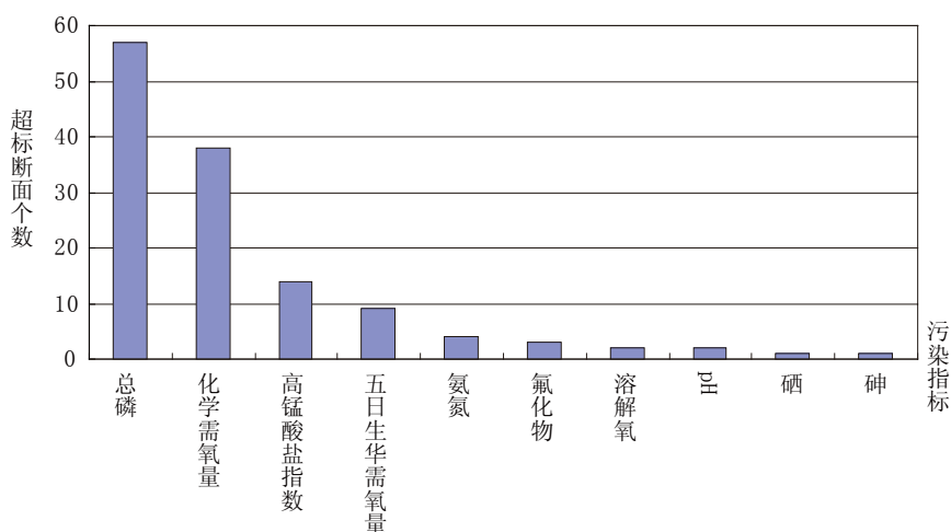
图1-4 2013年1月全国重点湖库污染指标统计
