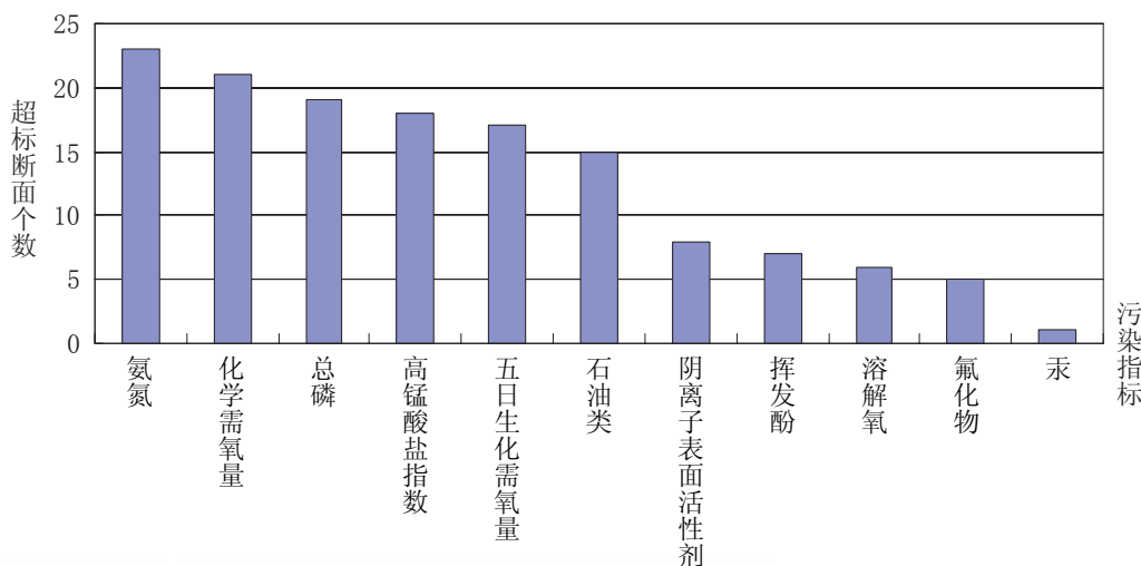
图2-11 海河流域水体污染指标统计
