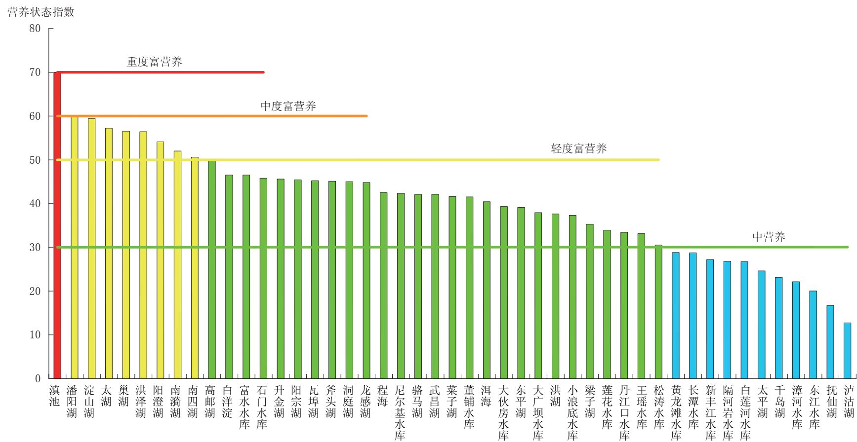
图 1-5 2013年1月全国重点湖库营养状态指数比较
