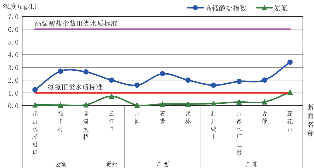
图2-6 珠江干流（西江）高锰酸盐指数、氨氮沿程变化
