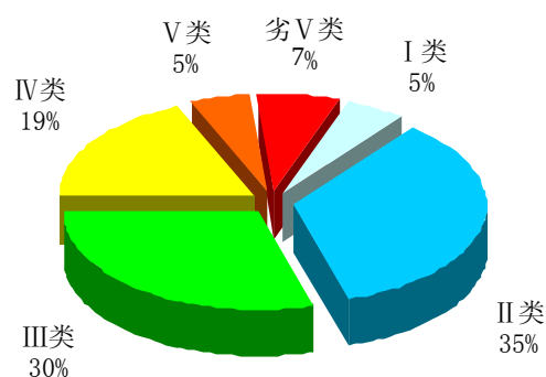
图2-3 2006年7月三峡库区及其上游水质类别比例
