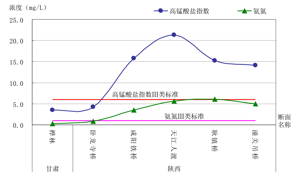
图 2-5 渭河高锰酸盐指数、氨氮浓度沿程变化
