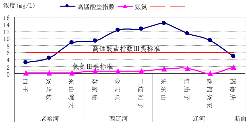
图 2-9 辽河干流高锰酸盐指数、氨氮浓度沿程变化
