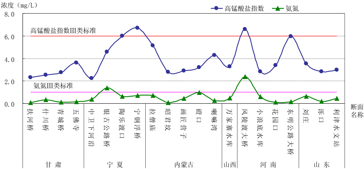
图 2-4 黄河干流高锰酸盐指数、氨氮浓度沿程变化
