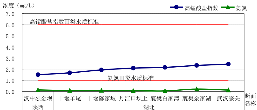
图2-2 汉江高锰酸盐指数、氨氮沿程变化
