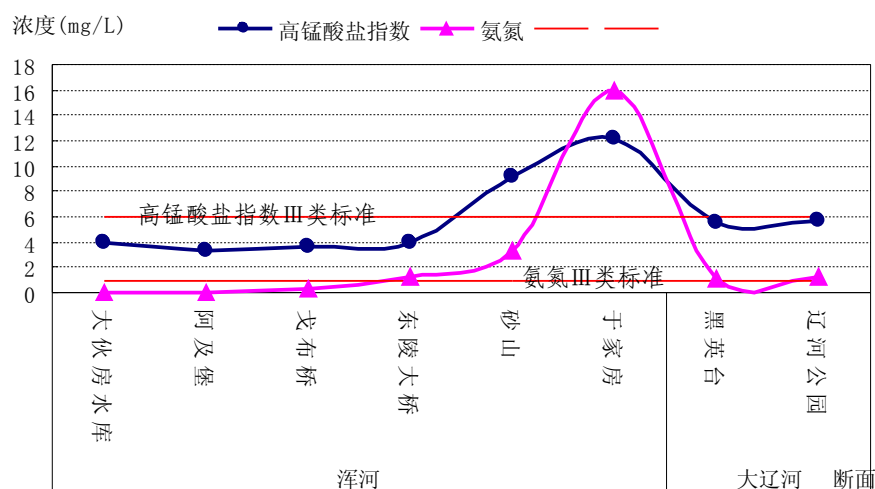
图 2-10 浑河、大辽河高锰酸盐指数、氨氮浓度沿程变化
