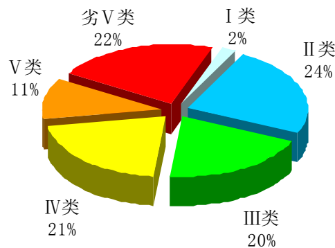
图 1-1 2006 年 7 月七大水系水质类别比例
