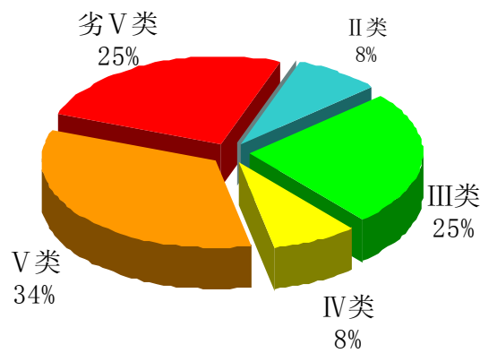
图 3-3 巢湖环湖河流水质类别比例
