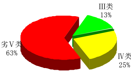
图 3-2 滇池环湖河流水质类别比例
