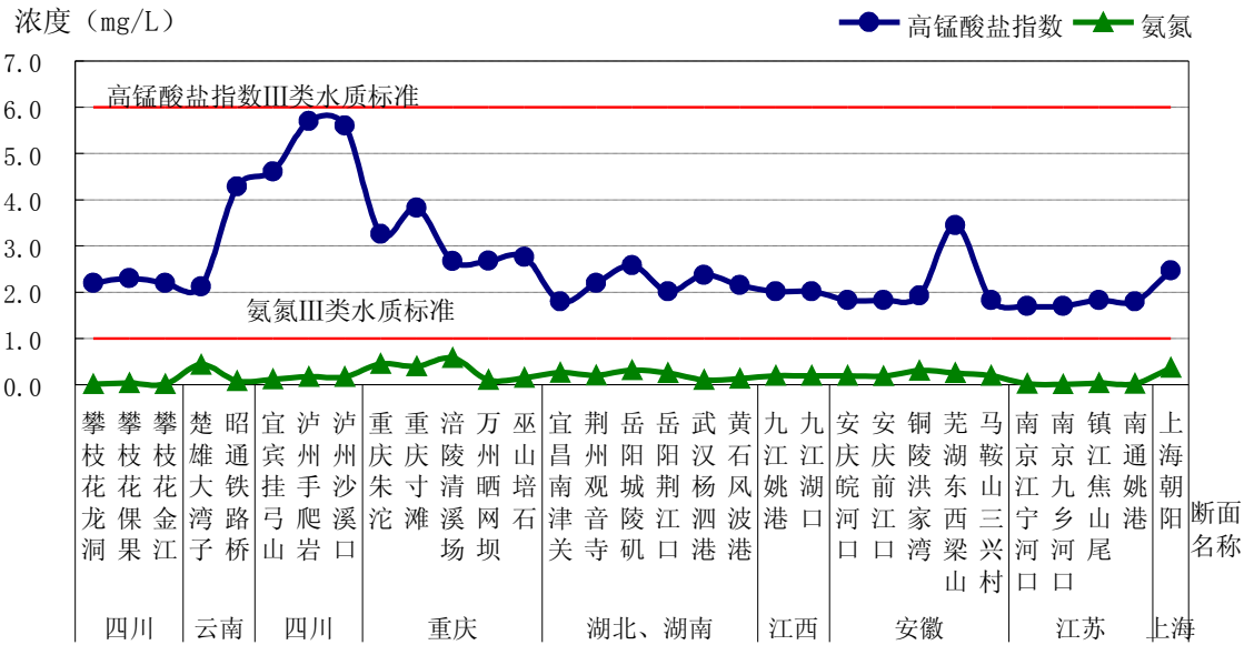
图2-1 长江干流高锰酸盐指数、氨氮沿程变化
