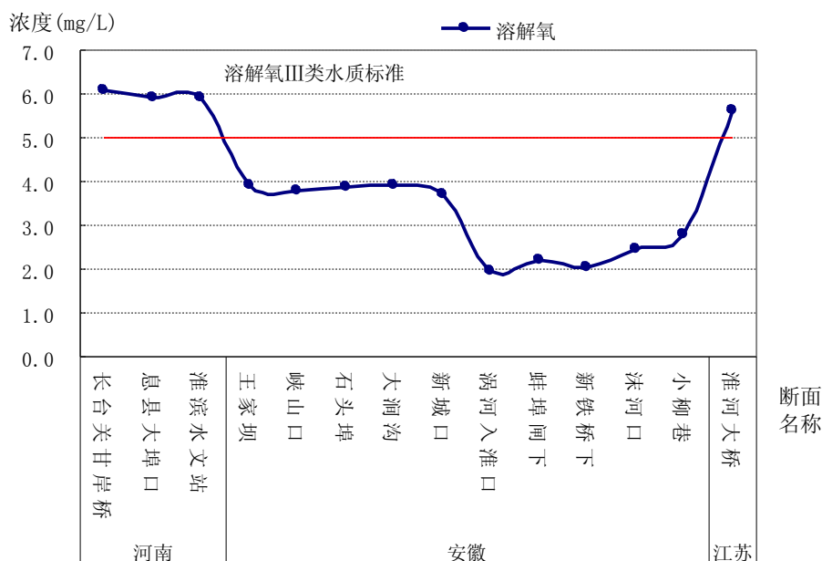
图 2-8 淮河干流溶解氧浓度沿程变化
