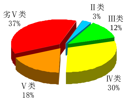
图 3-1 太湖环湖河流水质类别比例
