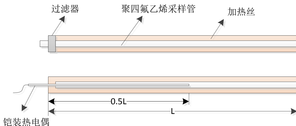
图5 采样管结构及测试方案示意图
