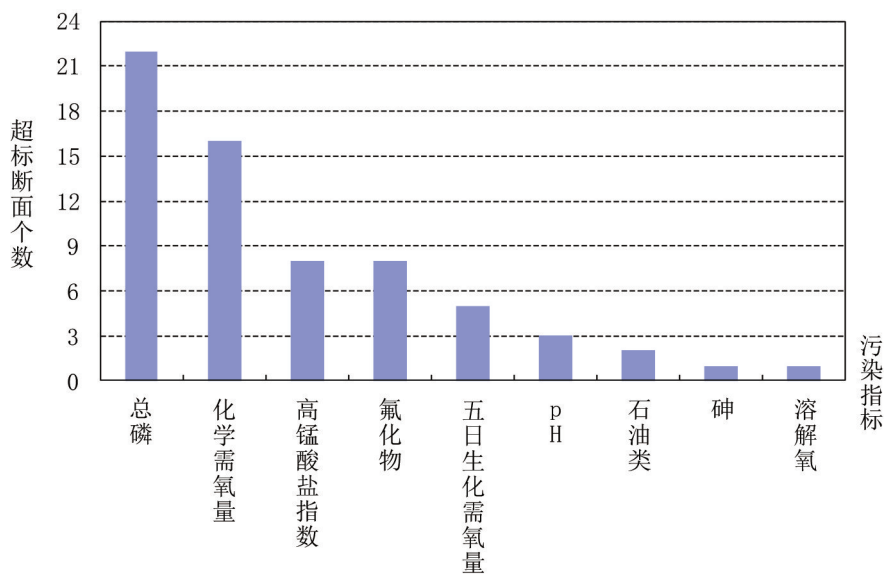
图1-4 2016年6月全国重点湖库污染指标统计
