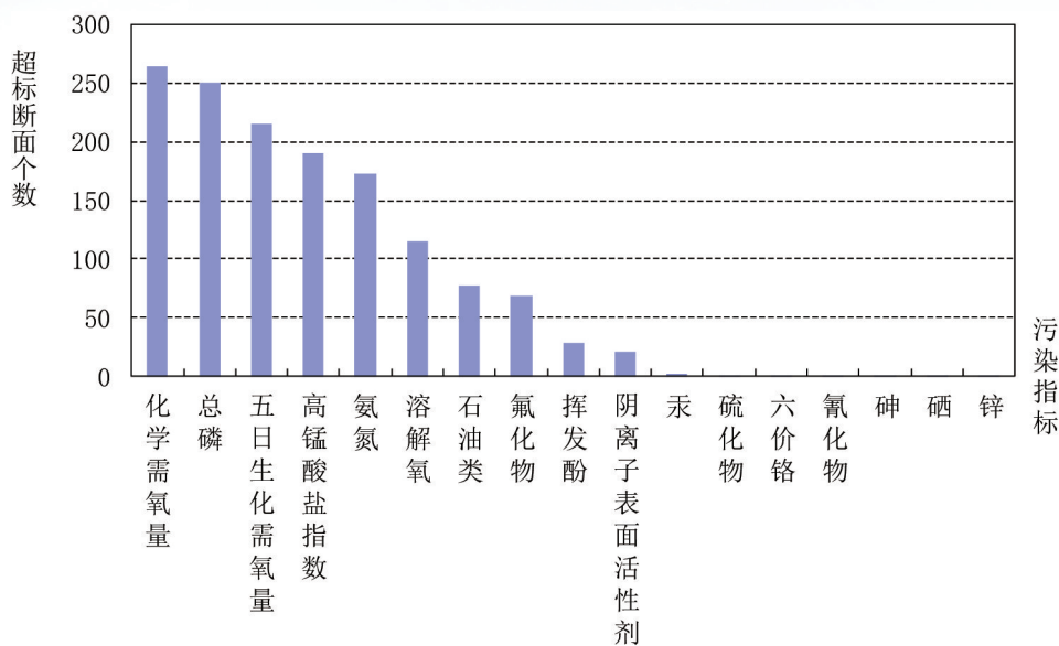
图1-2 2016年6月全国主要江河水系污染指标统计
