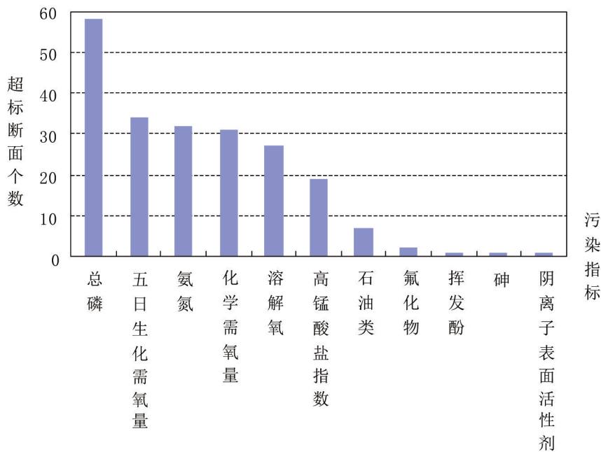
图 2-1 长江流域水体污染指标统计
