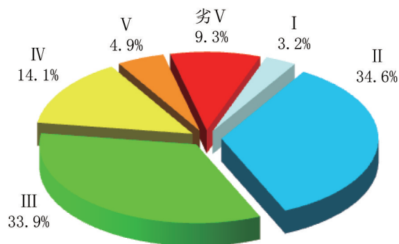
图 1-1 2016 年 6 月全国主要江河水系水质类别比例
