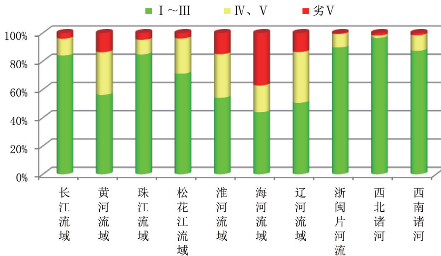
图1-3 2016年6月十大流域水质类别比例
