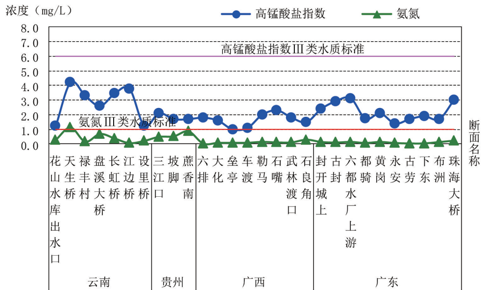
图2-6 珠江干流高锰酸盐指数、氨氮沿程变化
