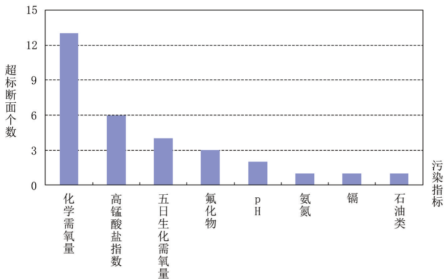
图 1-4 2016 年 4 月全国重点湖库污染指标统计
