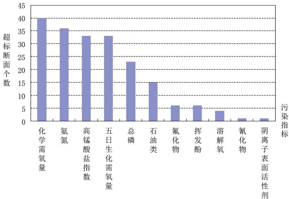
图2-12 辽河流域水体污染指标统计
