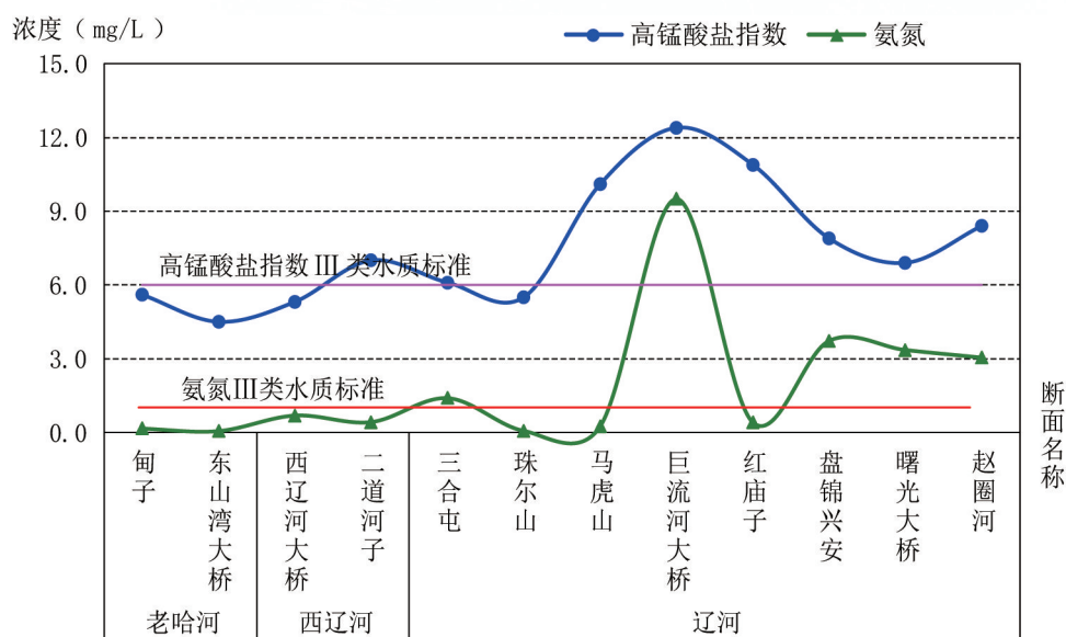
图2-13 辽河干流高锰酸盐指数、氨氮沿程变化
