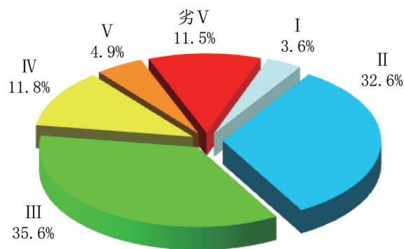
图1-1 2016年4月全国主要江河水系水质类别比例
