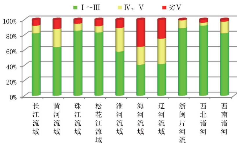
图 1-3 2016年4月十大流域水质类别比例
