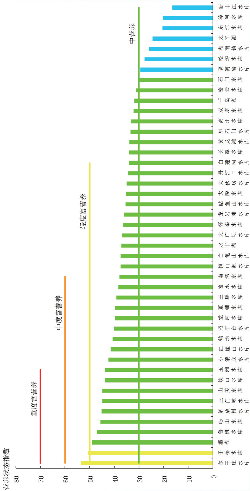
图 3-2 2016 年 4 月重要水库营养状态指数比较
