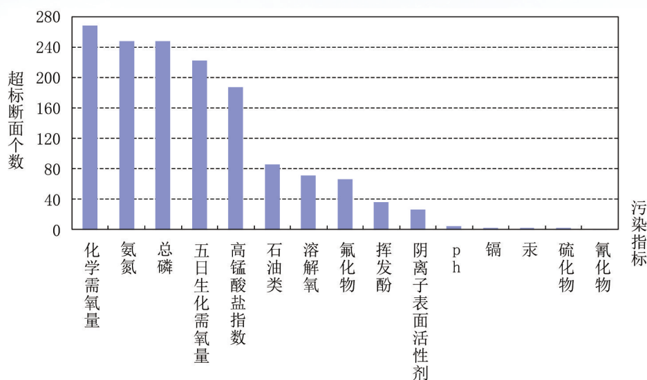
图 1-2 2016年4月全国主要江河水系污染指标统计
